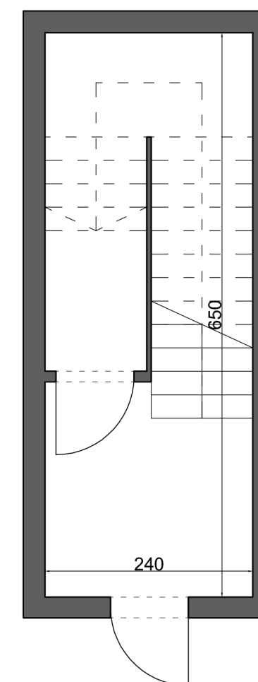
RZUT PARTERU
