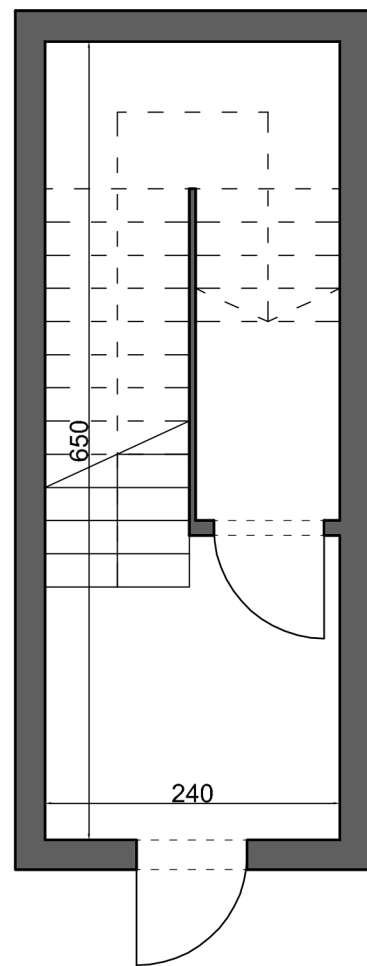
RZUT PARTERU
